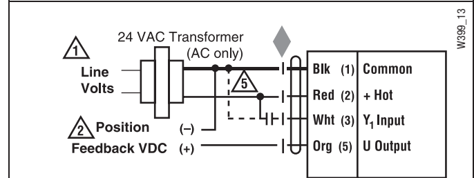
PWM
