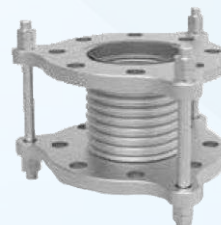
Khớp nối giãn nở linh hoạt Inox nối hàn Size: DN25 ~ DN400 | Thân: Inox (STS) Áp lực: 1.0 MPa/2.0 MPa | Nhiệt độ: <220°C/< 250°C
