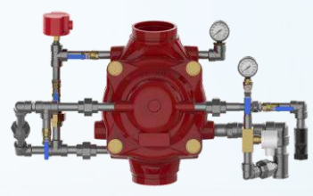
Van xả trần loại phản ứng nhanh nổi cùm KFI Product | Kích thước: DN80 – DN150 Thân: Gang | Áp lực max: 1.4 Mpa/2.2 Mpa
