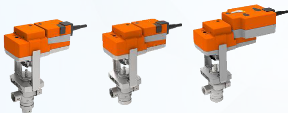
Van cầu 2 ngã/3 ngã điều khiển bằng điện nổi ren Loại điều khiển thường hoặc Fail-Safe | Điều khiển On-Off/3 điểm/Tuyến Tính Thân: Inox | Áp lực: PN25 | Nhiệt độ: 0°C ~ 130°C
