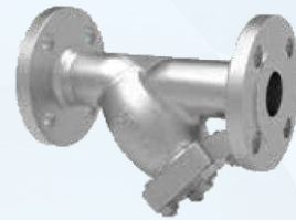
Y lọc bằng Gang nối ren/nối bích Size: DN15 ~ DN500 | Thân: Gang (GCD450) Áp lực max: 2.0 MPa | Nhiệt độ: <220°C
