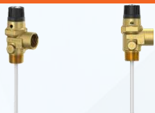
VAN AN TOÀN NHIỆT ÁP BẰNG ĐỒNG NỐI REN Áp lực max: 7Bar | Nhiệt độ: -10°C ~ 120°C
