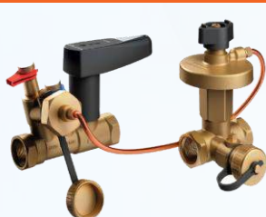
Van cân bằng chênh áp bằng Đồng nối ren Kích thước: DN15 ~ DN50 | Thân: Đồng/Gang Áp lực: PN16/PN25 | Nhiệt độ: -20°C ~ 120°C
