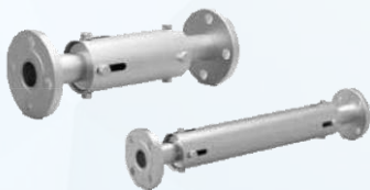
Khớp nối giãn nở Inox nối bích Size: DN25 ~ DN300 | Thân: Inox (STS) Áp lực max: 1.0 MPa | Nhiệt độ: <220°C
