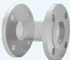
Khớp nối giãn nở linh hoạt Inox nối bích Size: DN25 ~ DN300 | Thân: Inox (STS) Áp lực: 1.0 MPa/2.0 MPa | Nhiệt độ: <220°C
