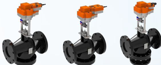
Van cầu 2 ngã/3 ngã điều khiển bằng điện nổi bích Loại điều khiển thường hoặc Fail-Safe | Điều khiển On-Off/3 điểm/Tuyến Tính Thân: Gang | Áp lực: PN16/PN25 | Nhiệt độ: 0°C ~ 150°C / 0°C ~ 180°C
