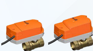
Zone Valve | Van vùng 2 ngã nổi ren Điều khiển On-Off/3 điểm/Tuyến Tính Thân: Đồng | Áp lực: PN25 | Nhiệt độ: 2°C ~ 100°C
