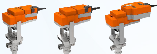
Van cầu 2 ngã/3 ngã điều khiển bằng điện nổi ren Loại điều khiển thường hoặc Fail-Safe | Điều khiển On-Off/3 điểm/Tuyến Tính Thân: Inox | Áp lực: PN25 | Nhiệt độ: 0°C ~ 130°C
