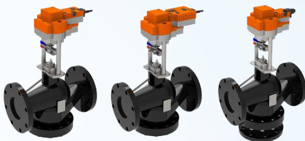
Van cầu 2 ngã/3 ngã điều khiển bằng điện nổi bích Loại điều khiển thường hoặc Fail-Safe | Điều khiển On-Off/3 điểm/Tuyến Tính Thân: Gang | Áp lực: PN16/PN25 | Nhiệt độ: 0°C ~ 150°C / 0°C ~ 180°C
