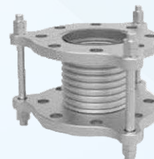
Khớp nối giãn nở linh hoạt Inox nối bích Size: DN25 ~ DN400 | Thân: Inox (STS) Áp lực: 1.0 MPa/2.0 MPa | Nhiệt độ: <220°C/< 250°C
