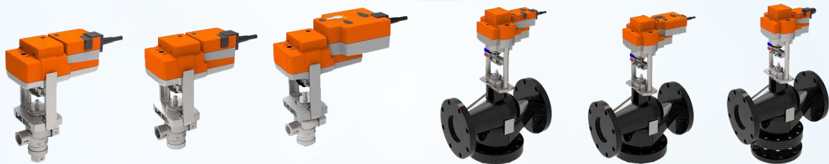
Van cầu 2 ngã/3 ngã điều khiển bằng điện nổi ren Loại điều khiển thường hoặc Fail-Safe | Điều khiển On-Off/3 điểm/Tuyến Tính Thân: Inox | Áp lực: PN25 | Nhiệt độ: 0°C ~ 130°C
